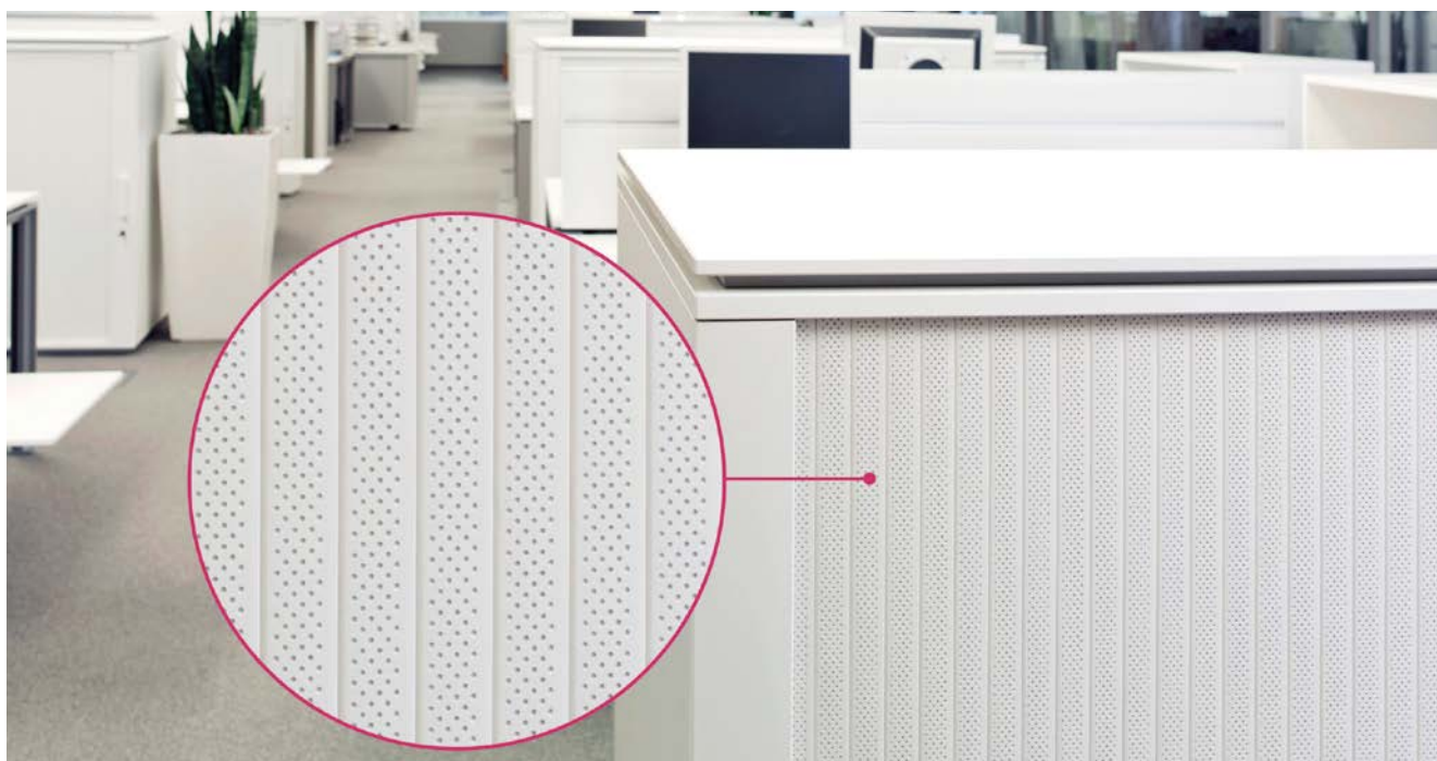
Az ISO 354 szabvány szerinti zajelnyelési terület (süllyesztett kamra) – szekrény előlapi felülettel 1,91 m 2
