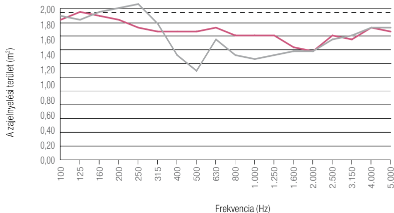
Az ISO 354 szabvány szerinti zajelnyelési terület (süllyesztett kamra) – szekrény előlapi felülettel 1,91 m 2
