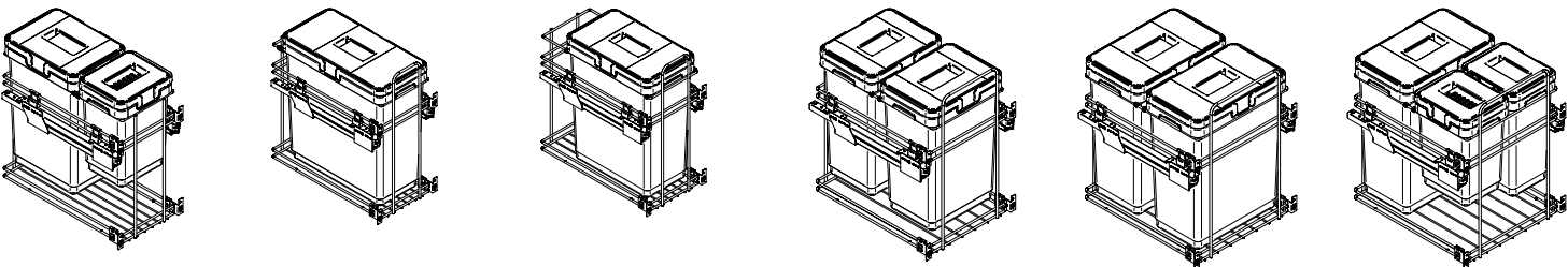
M 50 PKBGME502M (30+30) Lt M 50 PKBGME503M (30+10+9) Lt M 60 PKBGME602M (33+33) Lt M 60 PKBGME604M (20+20+10+9) Lt
