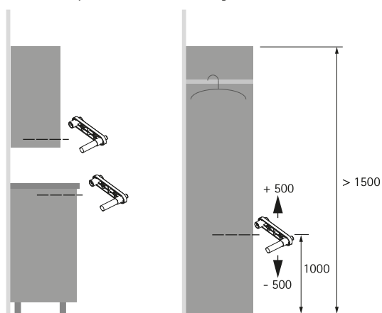
Magnetická aretace (provedení Standard a Design)
