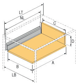
Frontkihúzású fiók, magassága 70/144 mm
