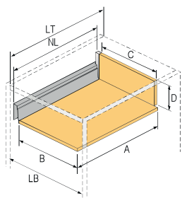
Frontkihúzású fiók, magassága 70/176 mm
