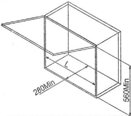
A. Upturn door structure
